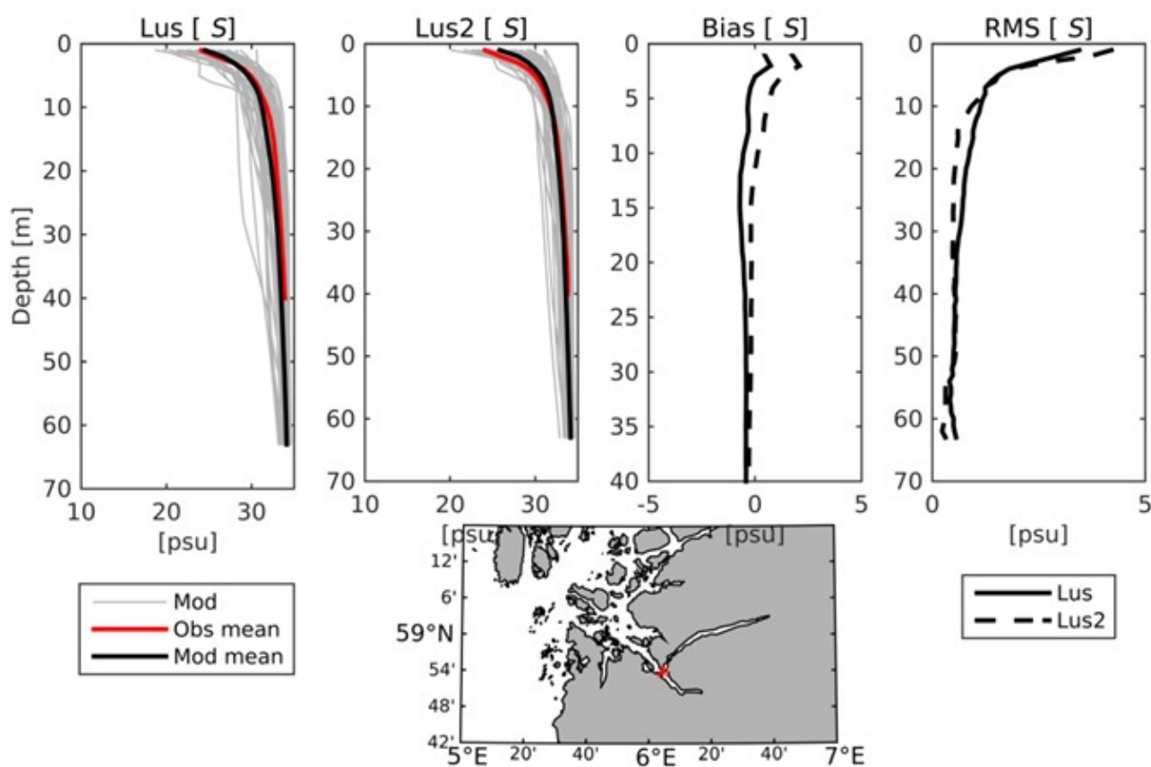
Figur 12. Øverst er vertikallprofiler av saltholdighet i Lus og Lus2 (venstre) og bias (modell – måling) og root-mean-square differanse (høyre). I venstre paneler viser grå linje alle modellprofiler i observasjonstidspunktene, svart linje viser middelprofilen fra modellen og rød linje viser middelprofilen fra observasjonene. I høyre paneler vises Lus som heltrukken linje og Lus2 som stiplet linje. Nederst er kart som viser stasjonens posisjon (rød stjerne).
