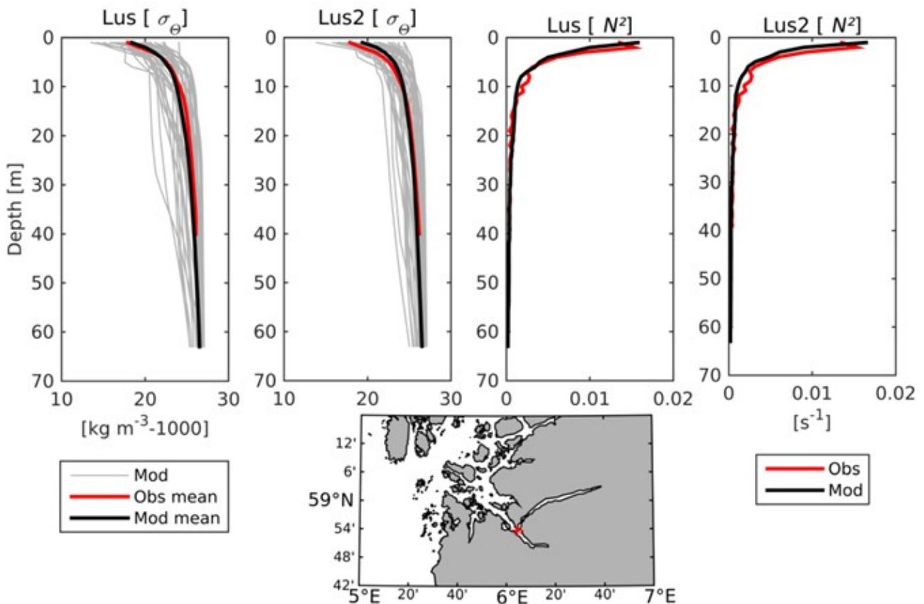
Figur 13. Samme som for Figur 12, men viser profiler for tetthetsanomali ( \text{kg m}^{-3} \cdot 1000 ; venstre) og Brunt-Väisälä frekvens ( \text{s}^{-1} ; høyre).
