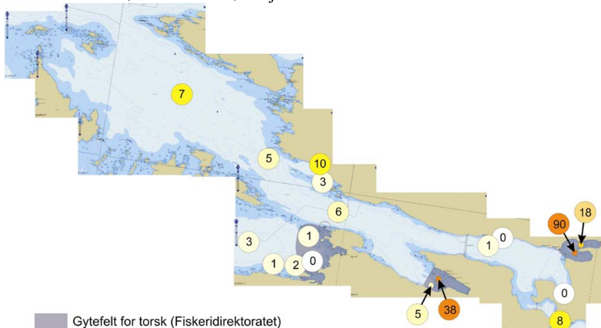
Figur 1. Stasjonsnett for eggprøver i Førdefjorden. Tall angir antall torskeegg i prøvene.
