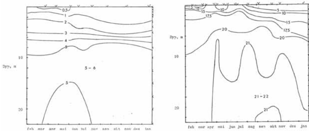
Figur 5. Totalt uorganisk karbon ( C_T ) i Sælenvannet i Hordaland sammenlignet med saltholdighet. Til venstre er C_T gitt i mmol/L i 1977; og til høyre saltholdighet i samme tidsrom (Børshheim 1979).
