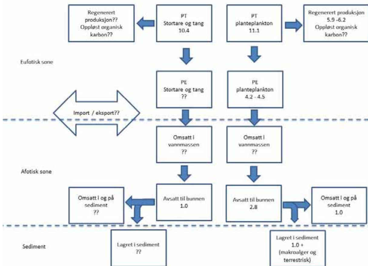
Figur 15. Tentativt karbonbudsjett til partikulært organisk karbon fra plateplankton og stortare og tang i kyst og fjord. Tall i millioner tonn. Tilførsel av terrestrisk partikulært organisk karbon (0.66), fra fiskeoppdrett (0.06) og fra industri (0.006) er ikke inkludert i figuren. PT = total primærproduksjon og PE = ny produksjon.
