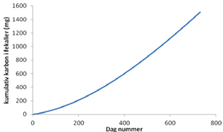
Figur 31. Modellert (DEB) produksjon av karbon i fekalier, uttrykt som mengde summert over tid (kumulativ) for et blåskjell som er 15 mm i skallengde og 50 mg i tørrvekt av bløtdeler ved dag 0 og 1000 mg i tørrvekt etter 2 år.
