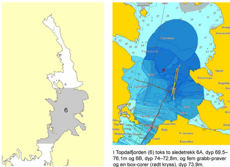
Figur 3.6. Topdalsfjorden 6
