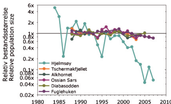
Figur 4.8.1.6 Utviklingen i hekkebestanden av polarlomvi på Hjelsmøya samt utvalgte lokaliteter på Svalbard vist som bestand (antall individer i prøvefelt) i prosent av gjennomsnitt for alle år den er overvåket. For en mer detaljert kartforklaring, se Figur 4.8.1.2.
