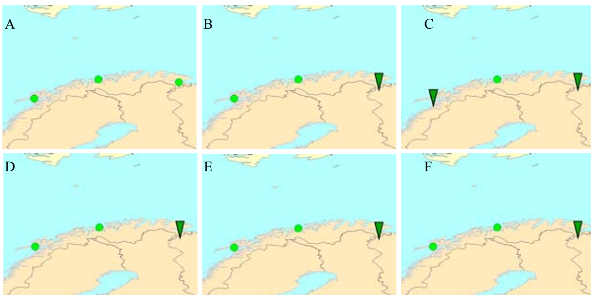
Figur 4.11.5.1. Trend 1992-2006 og konsentrasjon for 2006 i forhold til SFTs Klasse I for kadmium (A), kvikksølv (B), bly (C), PCB (D), DDT (E) og HCB (F) i torskelever eller torskemuskel (kvikksølv). Trekant opp/ned indikerer opp-/nedgående trend og sirkel indikerer ingen trend eller ikke tilstrekkelig data for å gjennomføre en trendanalyse. Rødt/grønt symbol betyr over/under øvre grense i SFTs Klasse I (Ubetydelig eller Lite forurensset).
