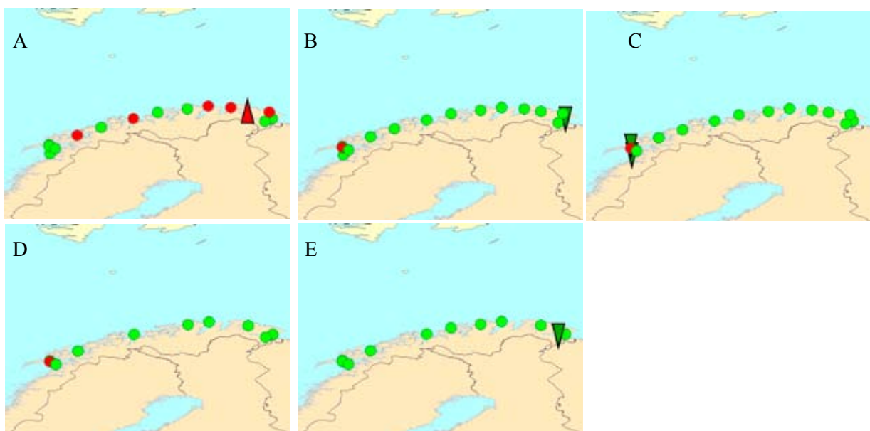
Figur 4.11.6.1 Trend 1992-2006 og konsentrasjon for 2006 i forhold til SFTs Klasse I for kadmium (A), kvikksølv (B), bly (C), PCB (D), DDT (E) og HCB (F) i blåskjell. Trekant opp/ned indikerer opp/nedadgående trend og sirkel indikerer ingen trend eller ikke tilstrekkelig data for å gjennomføre en trendanalyse. Rødt/grønt symbol betyr over/under øvre grense i SFTs Klasse I (Ubetydelig eller Lite forurenset).
