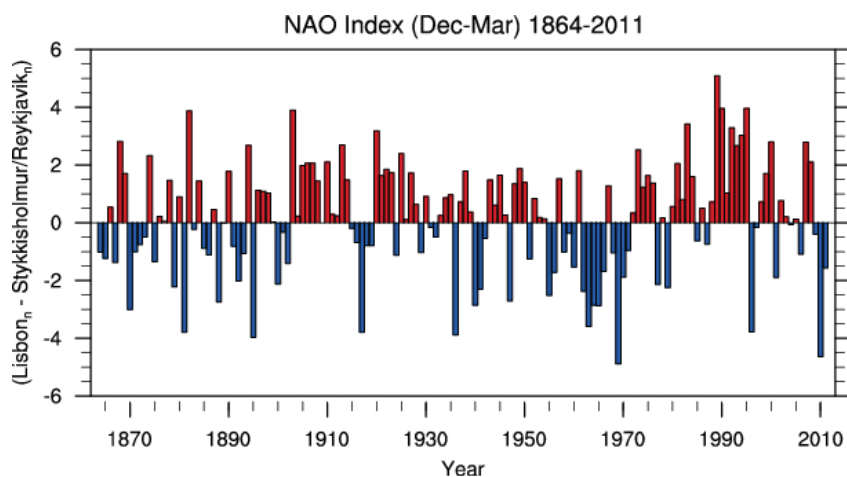
Figur 3. Tidsserie av vinterverdier (Desember-Mars) av den nordatlantiske oscillasjon (NAO) indeksen ( http://www.cgd.ucar.edu/cas/jhurrell/nao.stat.winter.html ).
