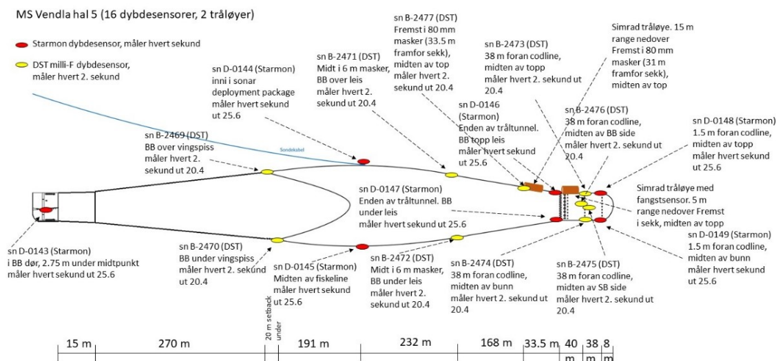
Figur 20. Trålinstrumentering, hal 5
