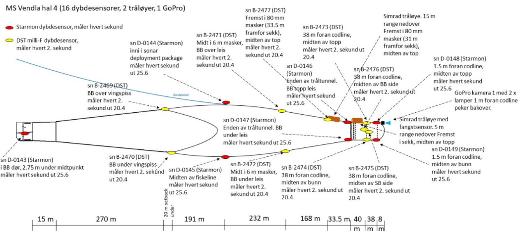
Figur 16. Trålinstrumentering, hal 4
