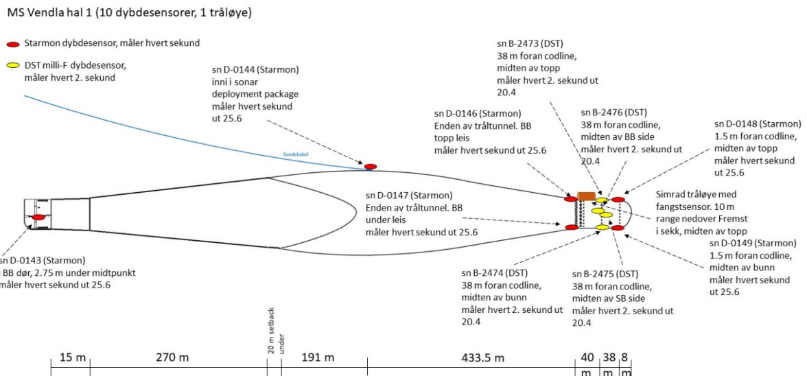
Figur 9. Trålinstrumentering, hal 1
